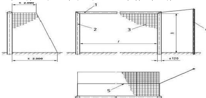
Σχ. Εστία ποδοσφαίρου Τύπου 1 (EN 748: 2013)
